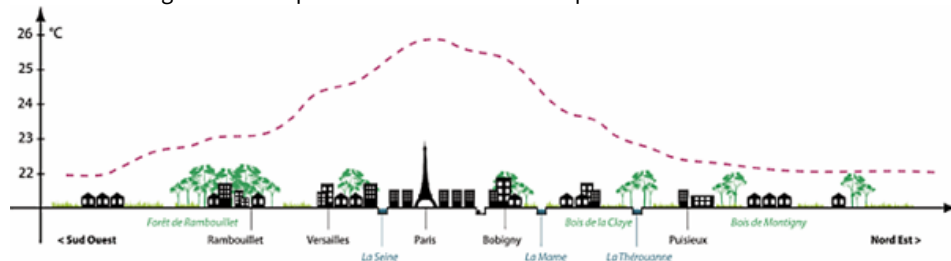
Fig 18 - Schématisation d'un îlot de chaleur urbain, d'après La Consultation internationale « le Grand Pari(s) de l'agglomération parisienne », Groupe Descartes, 2009 12 .
